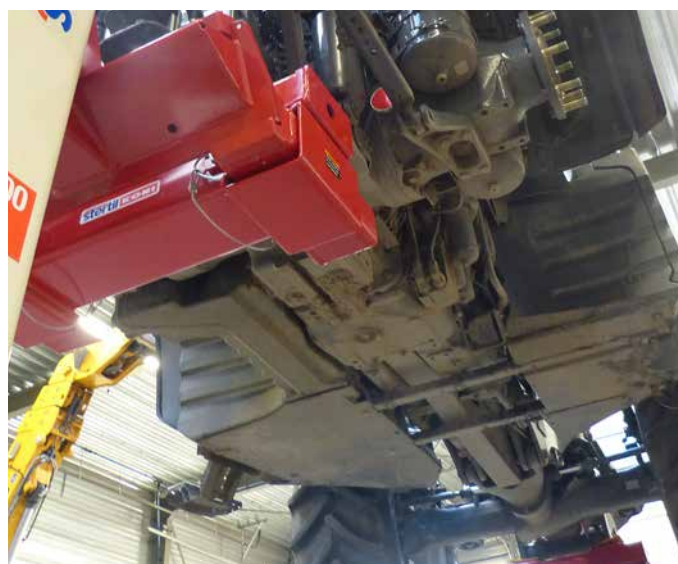
Specjalne adaptory podnoszące do podnoszenia wolnego od kół.
