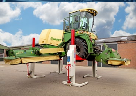
PRZESTAWNY PODNOŚNIK KOLUMNOWY
